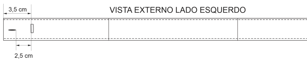
Figura 5 – Detalhes do posicionamento do gancho de alfaite no córs (Tolerância \pm 0,5\text{cm} ) Medidas em cm
