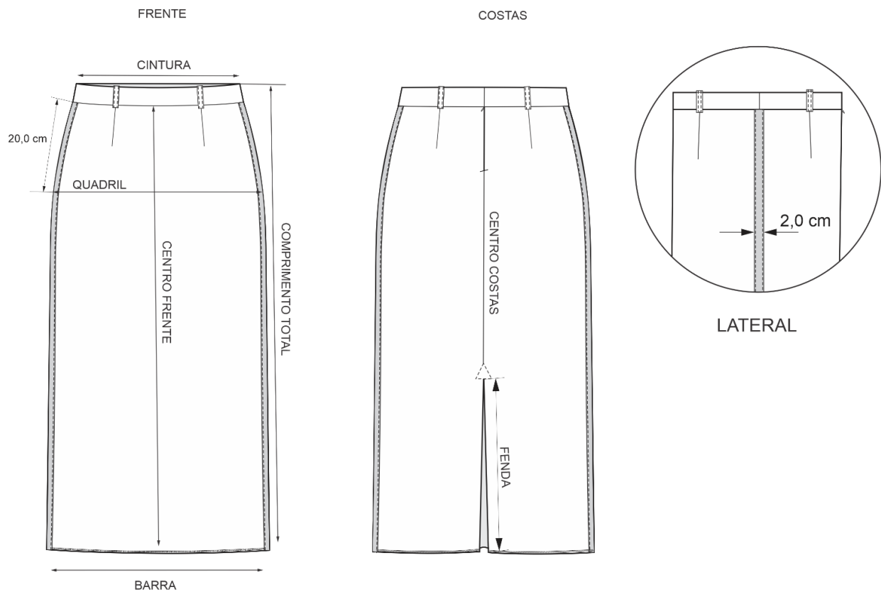
Figura 2 – Detalhes das medidas básicas frente e costas - Saia Longa
