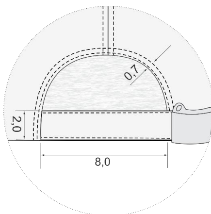
Figura 7 – Detalhes da abertura traseira do Gorro de Prontoidão
