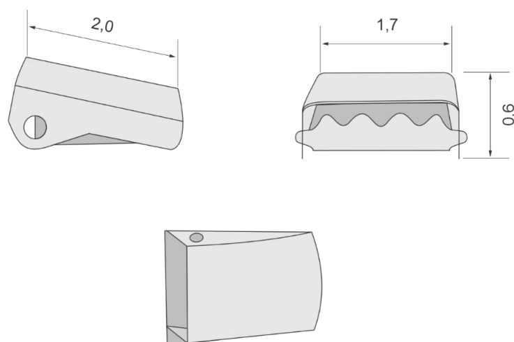
Figura 9 – Fivela de fechamento do Gorro de Prontoidão
