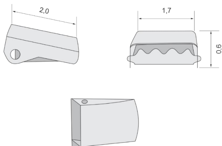
Figura 9 – Fivela de fechamento do Gorro de Prontidão Medidas em cm
