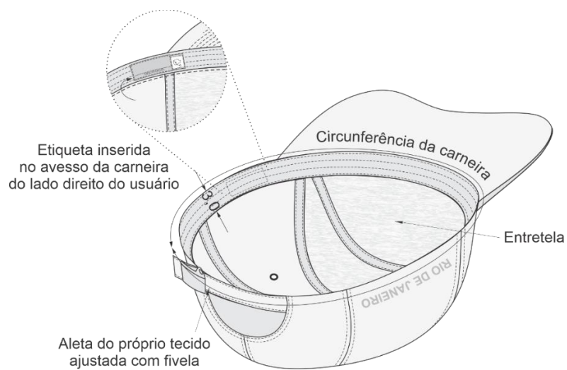
Figura 6 – Vista lateral do Gorro de Prontidão
