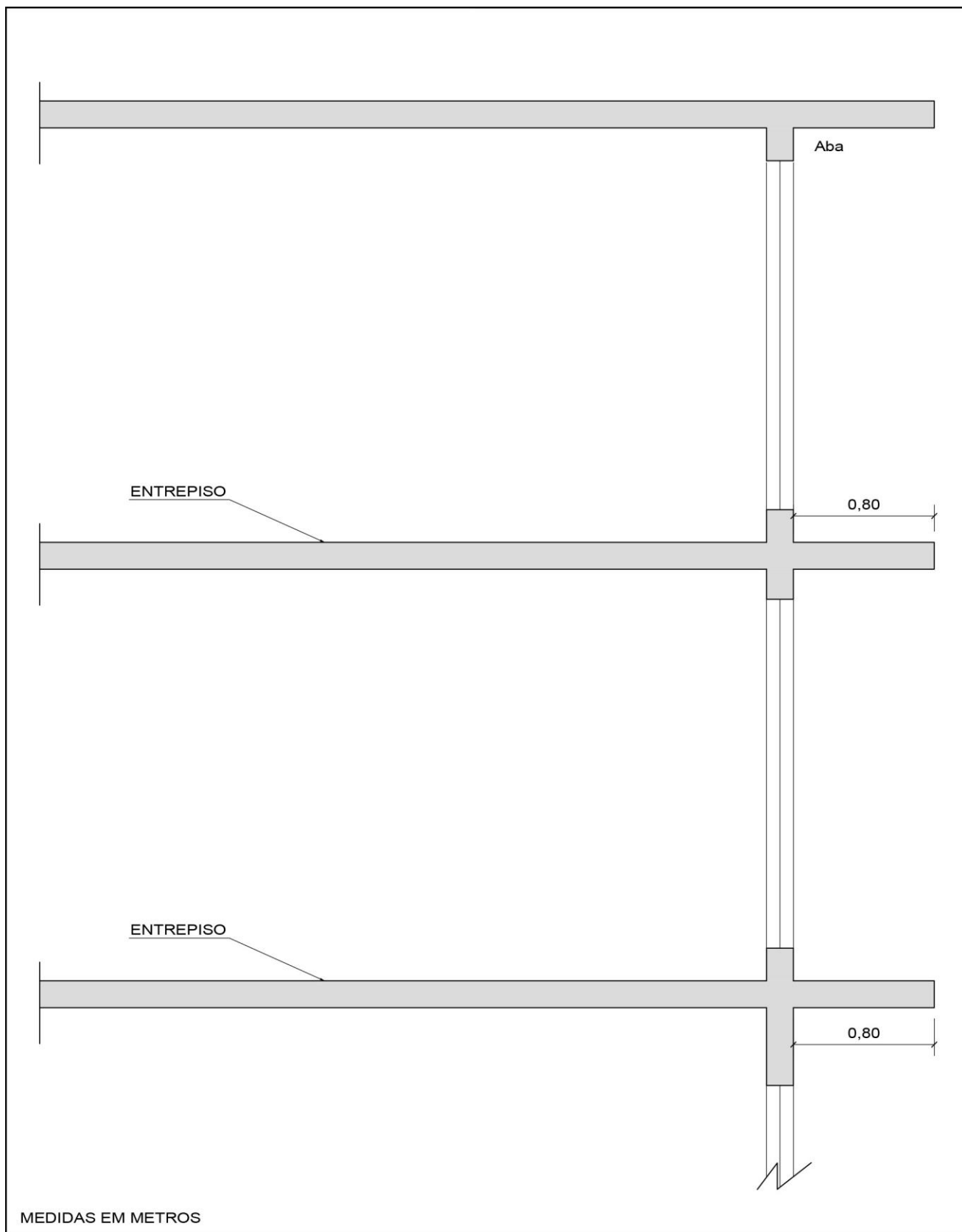
Figura 2: Modelo de compartimentação vertical (beiral)
