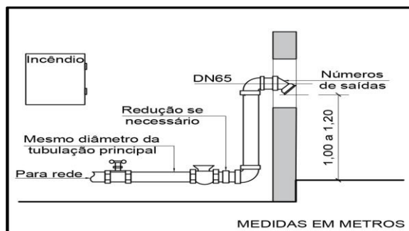
Figura 1: Dispositivo de recalque tipo coluna
