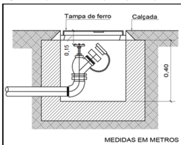
Figura 2: Dispositivo de recalque no passeio público
